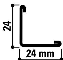
L24x24 C
